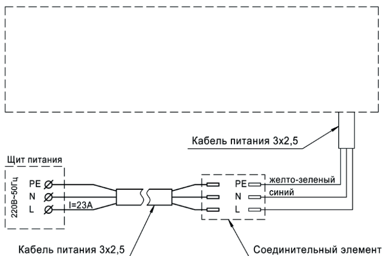
Рис. 2 Схема подключения завесы LTZR-5.0 S
